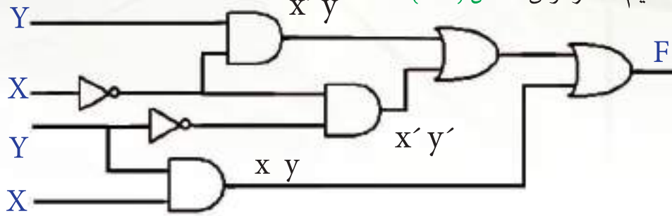
شكل (٨-١) دائرة تنظيم البوابات المنطقية للدالة: F = x' \times y' + x \times y' + x \times y
