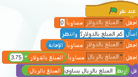
شكل (٢-٦-١): المقطع البرمجي للتحويل من الدولار إلى الريال
