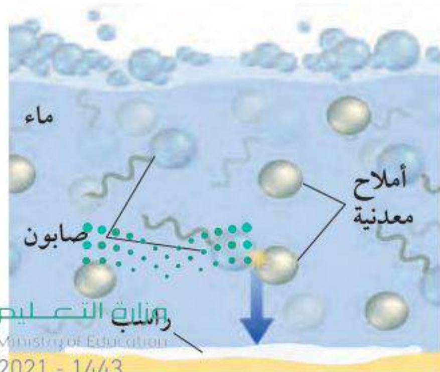
الشكل ٣ تتفاعل الأملاح مع الصابون فتشكل راسبًا.
